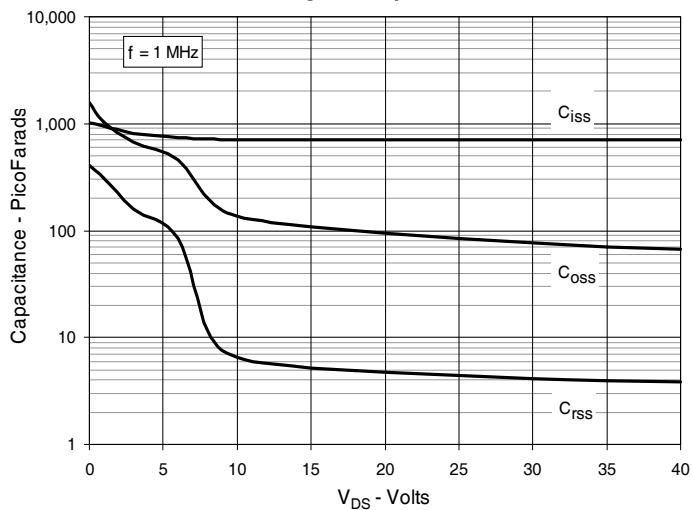
Fig. 11. Capacitance
