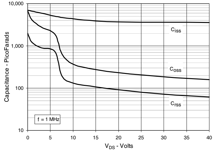
Fig. 14. Capacitance
