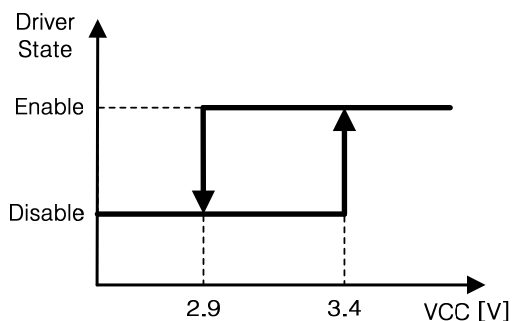
Figure 28. UVLO
