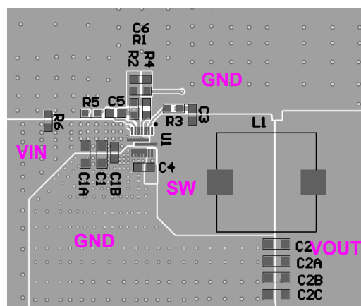
Top Layer
