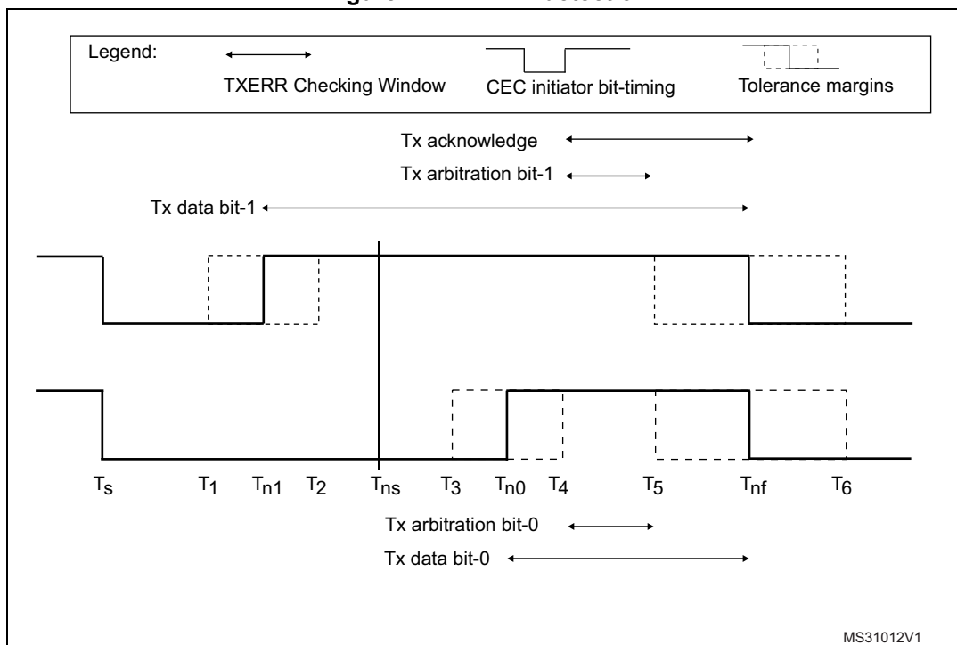
Figure 411. TXERR detection
