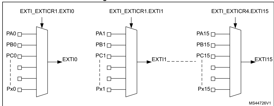
Figure 27. EXTI GPIO mux
