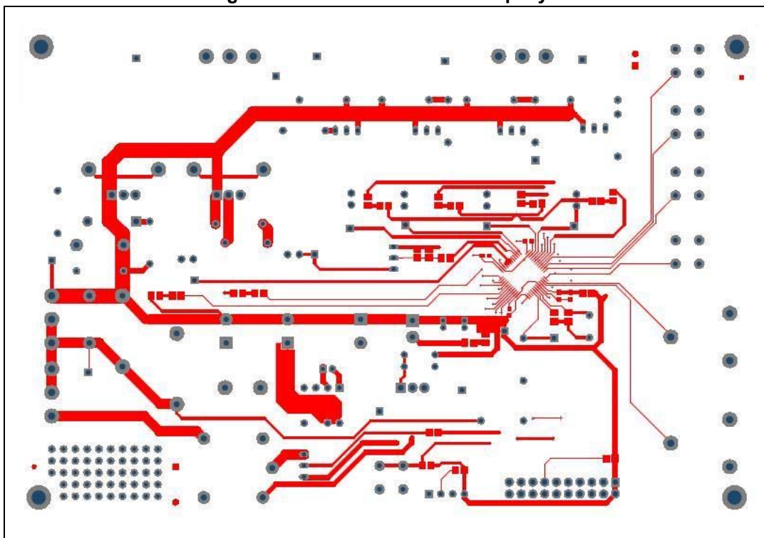
Figure 10. STEVAL-IHT005V2 - top layer
