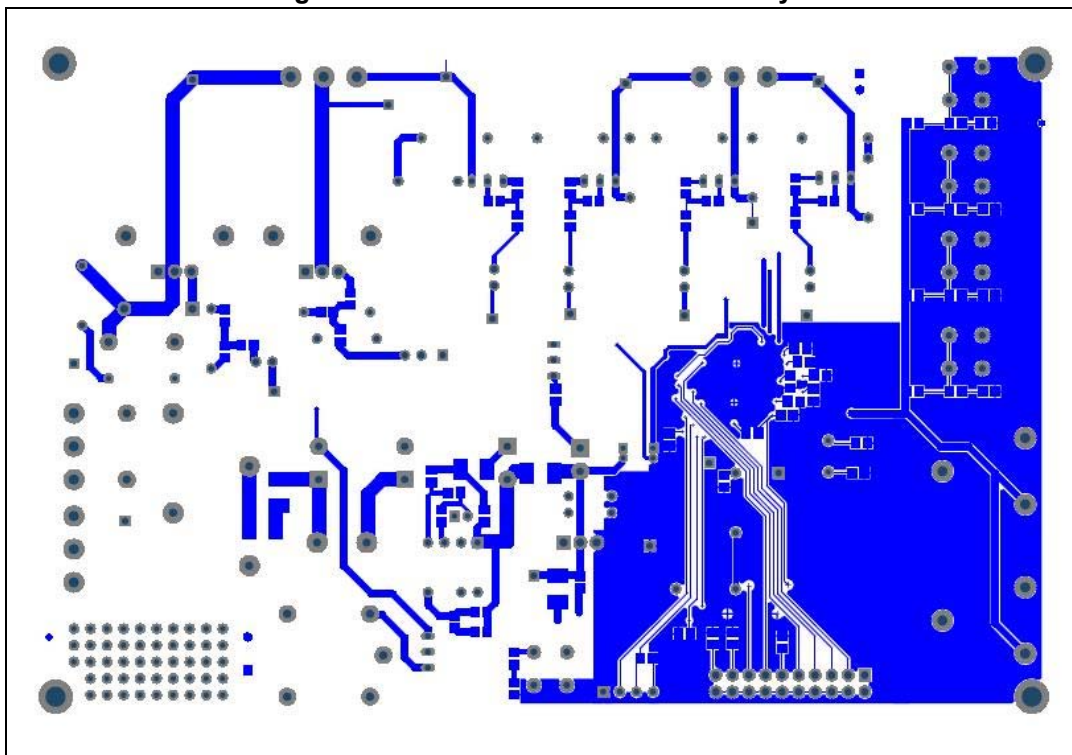
Figure 11. STEVAL-IHT005V2 - bottom layer
