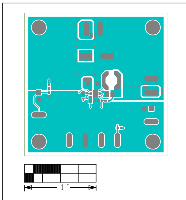
MAX17671F EV Kit—Top Layer
