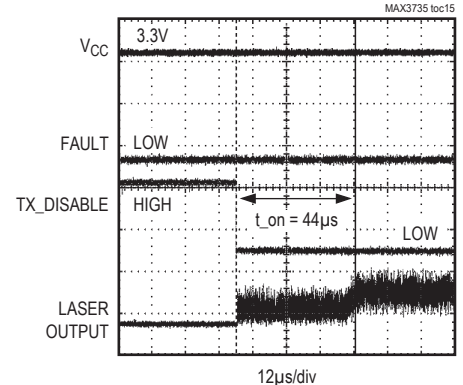
TRANSMITTER ENABLE
