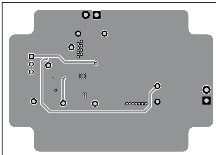
Figure 17. Bottom Layer
