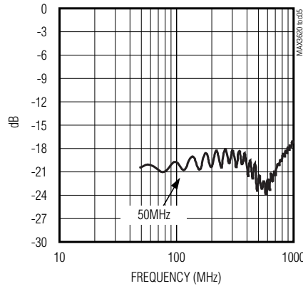
MAX3620A S11
