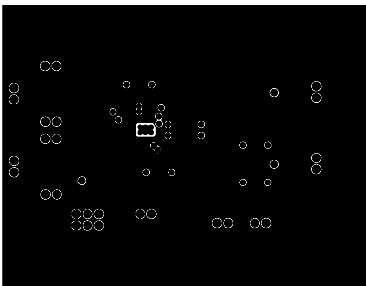
Figure 34. Bottom Layer
