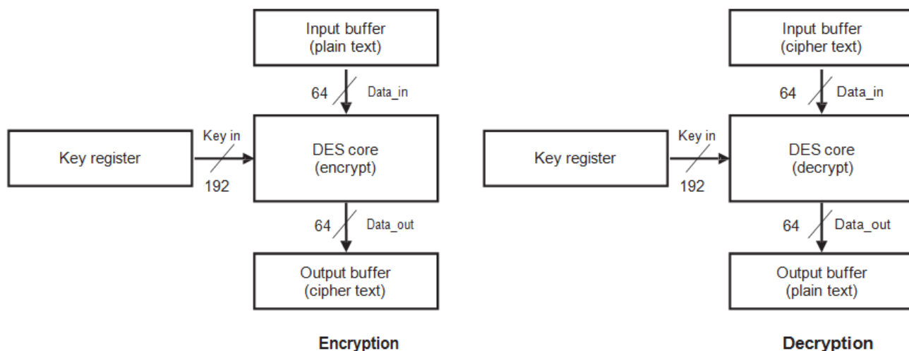
Figure 18-2. DES – ECB Feedback Mode
