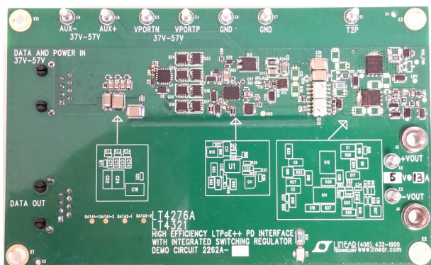
Top Side
