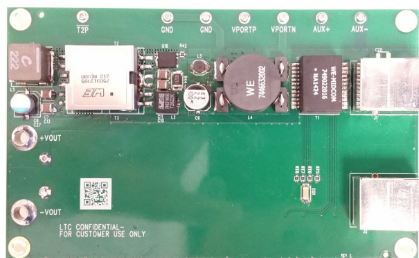
Bottom Side
