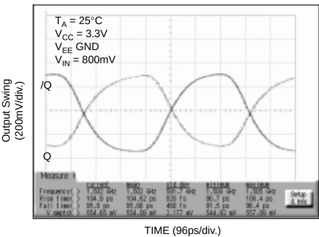
1.5GHz Output
