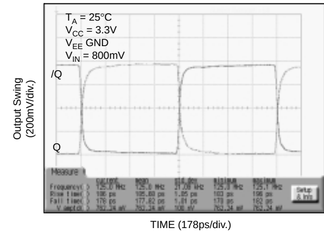
125MHz Output
