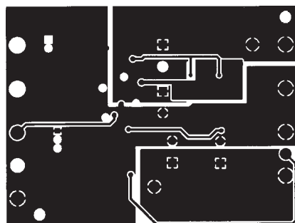
Copper Layer 3
