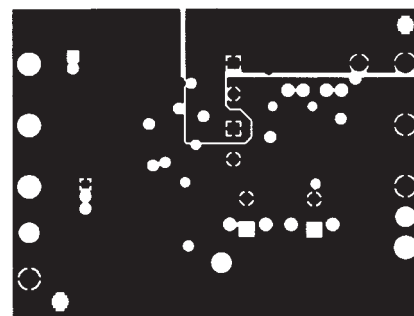
Copper Layer 2
