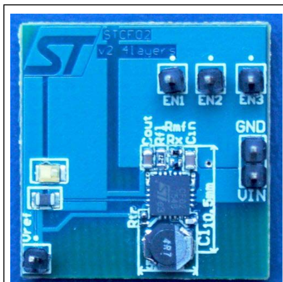
STEVAL-TLL003V1
