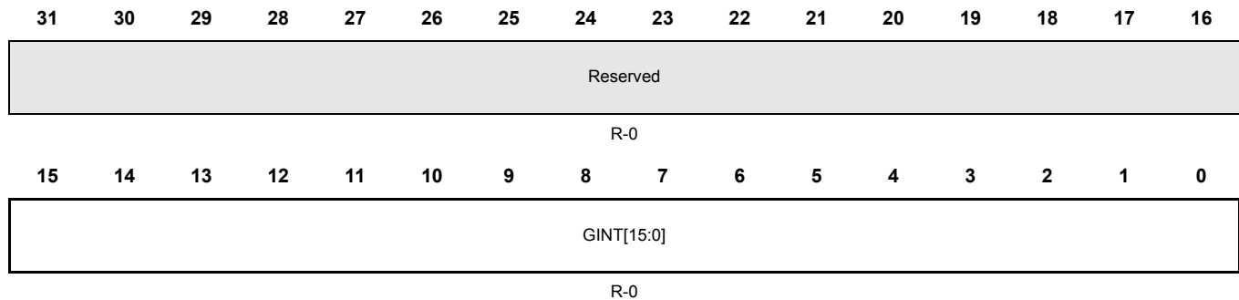
Figure 20-49. Global Interrupt Flag Register (GINTFLAG) [offset = 0x11C]
