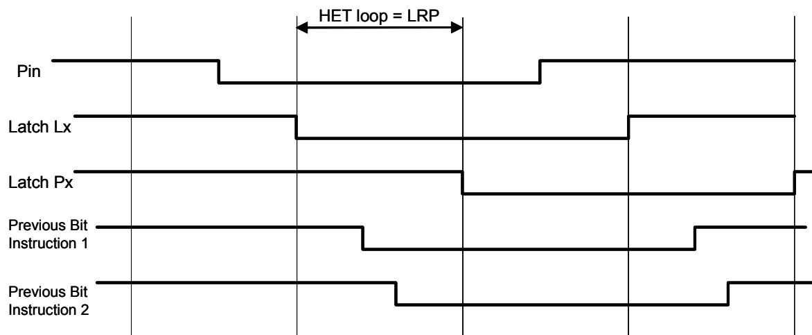
Figure 18-18. Edge Detection
