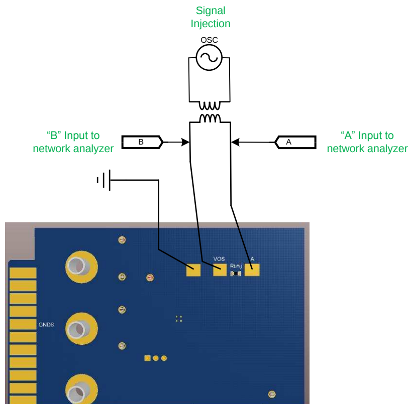
Figure 4. FRA Set-up
