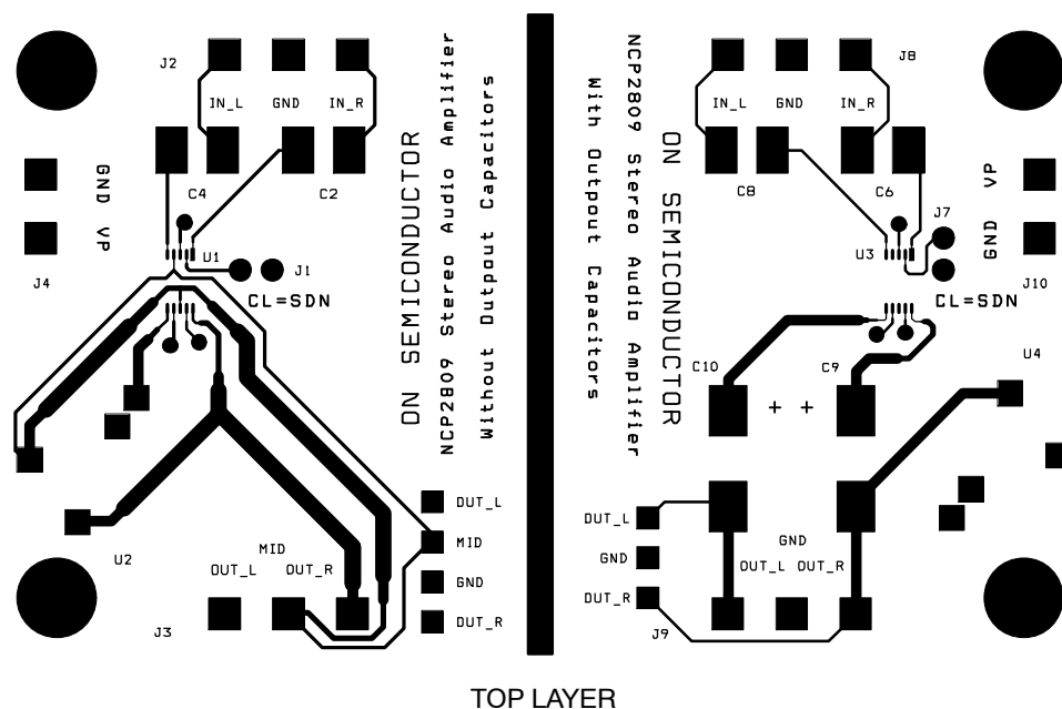
TOP LAYER
