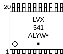
TSSOP-20
