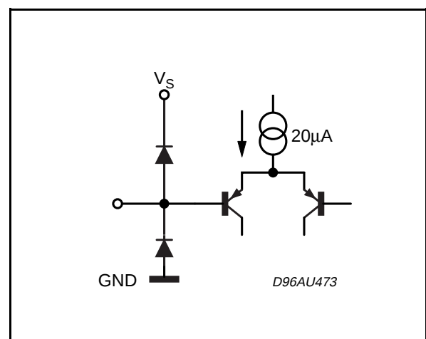
PIN: NETW2
