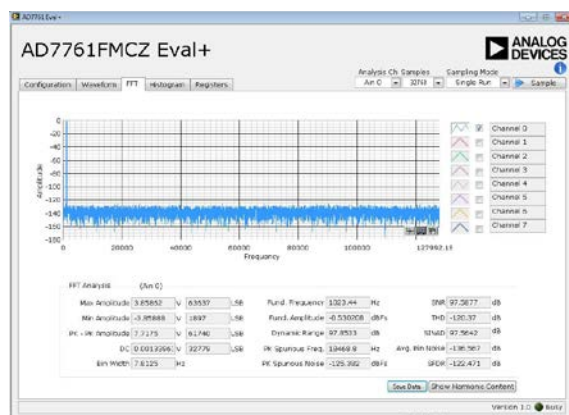
Figure 20. FFT Tab
