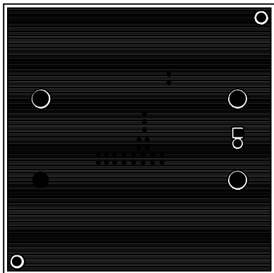
Layer 4, Solder Side*
