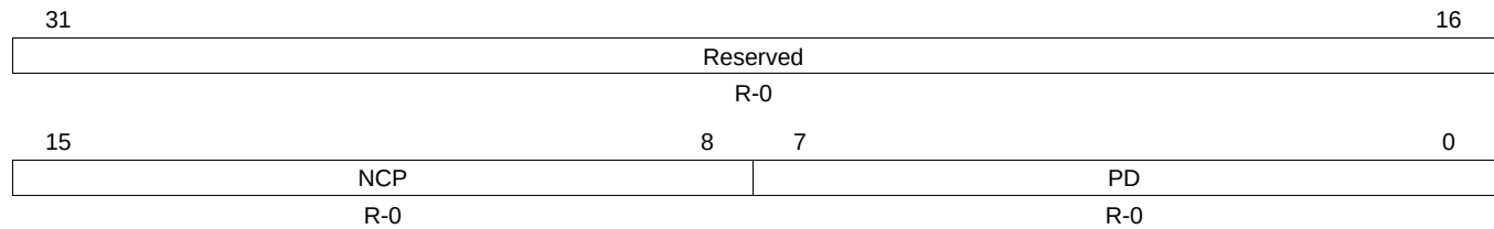
Figure 29-8. BIST Active FIS Register (BISTAFR)
