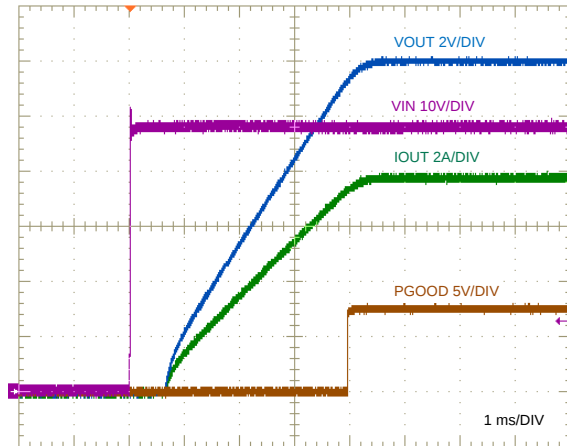
V_{IN} step to 48 V 1.5- \Omega Load
