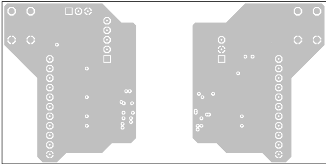
Inner Layer 1
