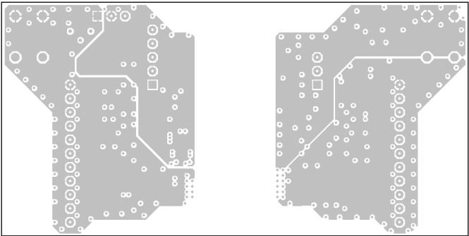
Inner Layer 2
