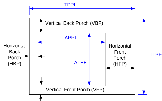
Figure 26. Timing Parameter Diagram
