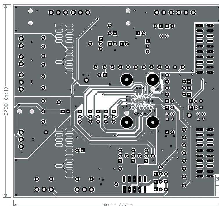
Figure 25. Bottom Layer
