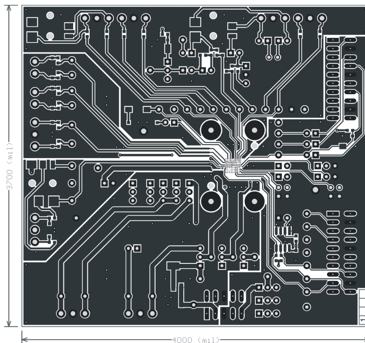
Figure 22. Top Layer
