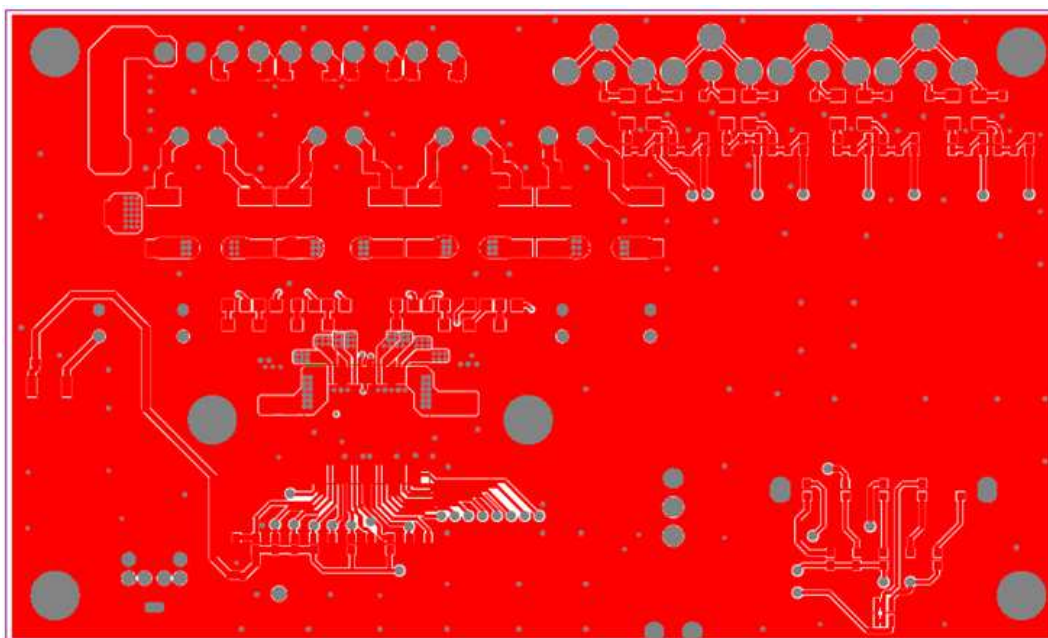
Figure 19. TAS5424CDKD Top Layer
