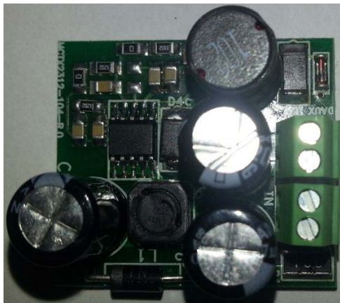
STEVAL-ISA115V1
