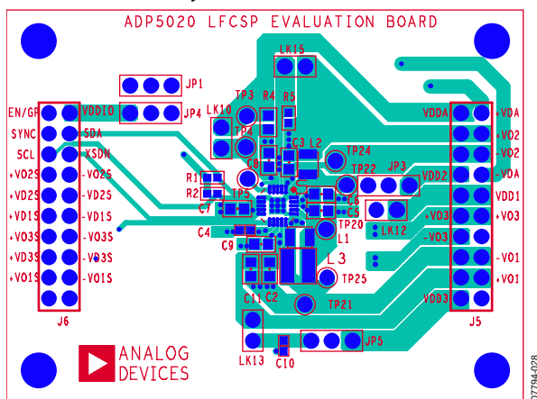
Figure 28. Top Layer
