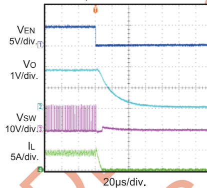
Enable Shut-down
