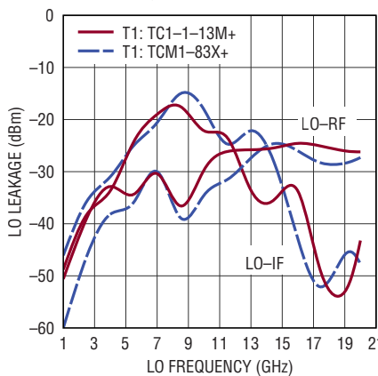
LO Leakage
