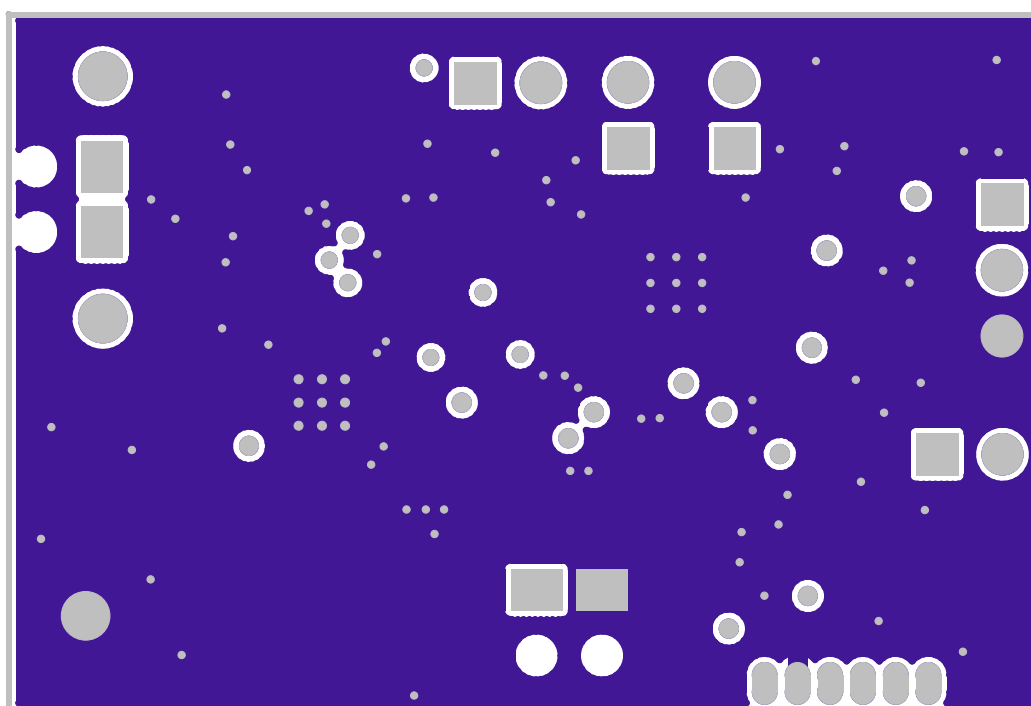
Figure 20. EVM Bottom Layer
