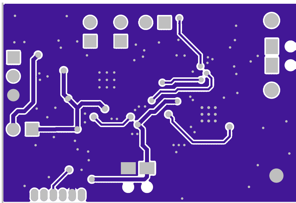
Figure 19. EVM Layer 3
