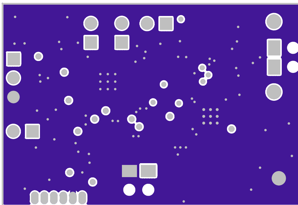
Figure 18. EVM Layer 2
