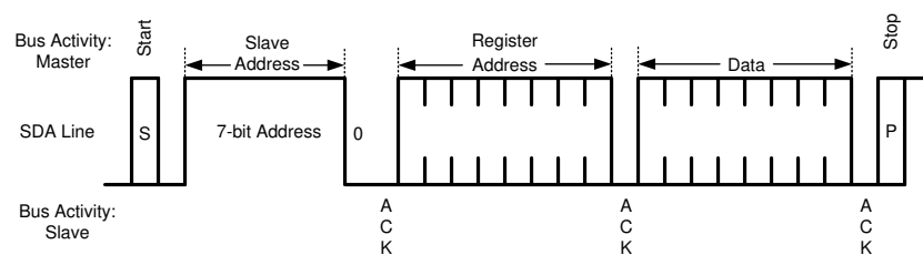
Figure 21. Write Byte
