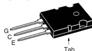
PLUS247 (IXBX)
