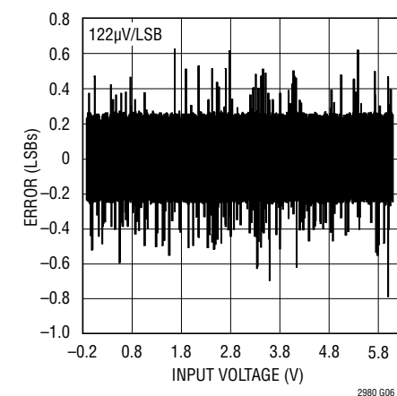
ADC DNL
