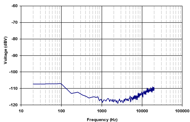
NOISE FFT
