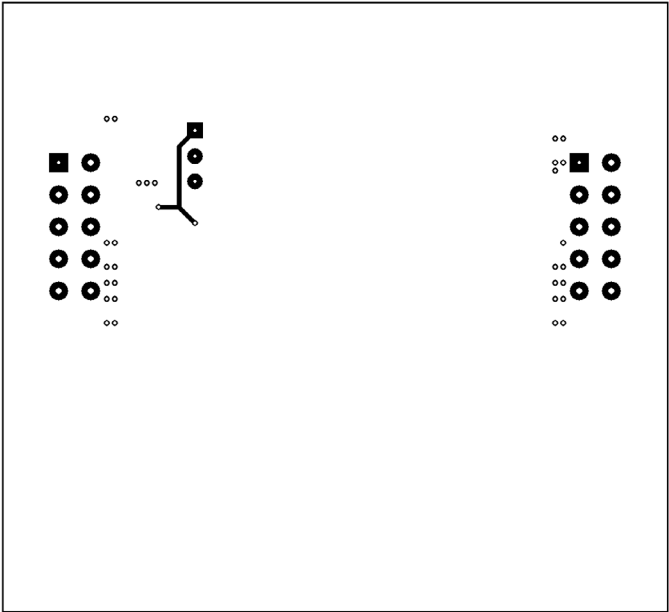
Layer 3. Signal Layer
