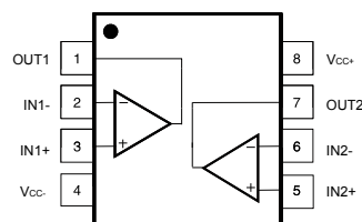
MiniSO8/SO8
