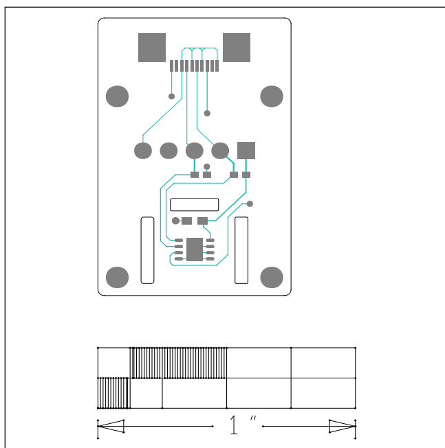
MAX30205 EV—Top
