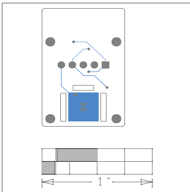
MAX30205 EV—Bottom
