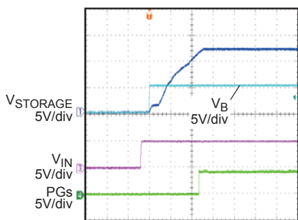
V_{STORAGE} Charge
