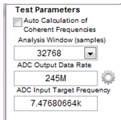
Figure 29. Test Parameters
