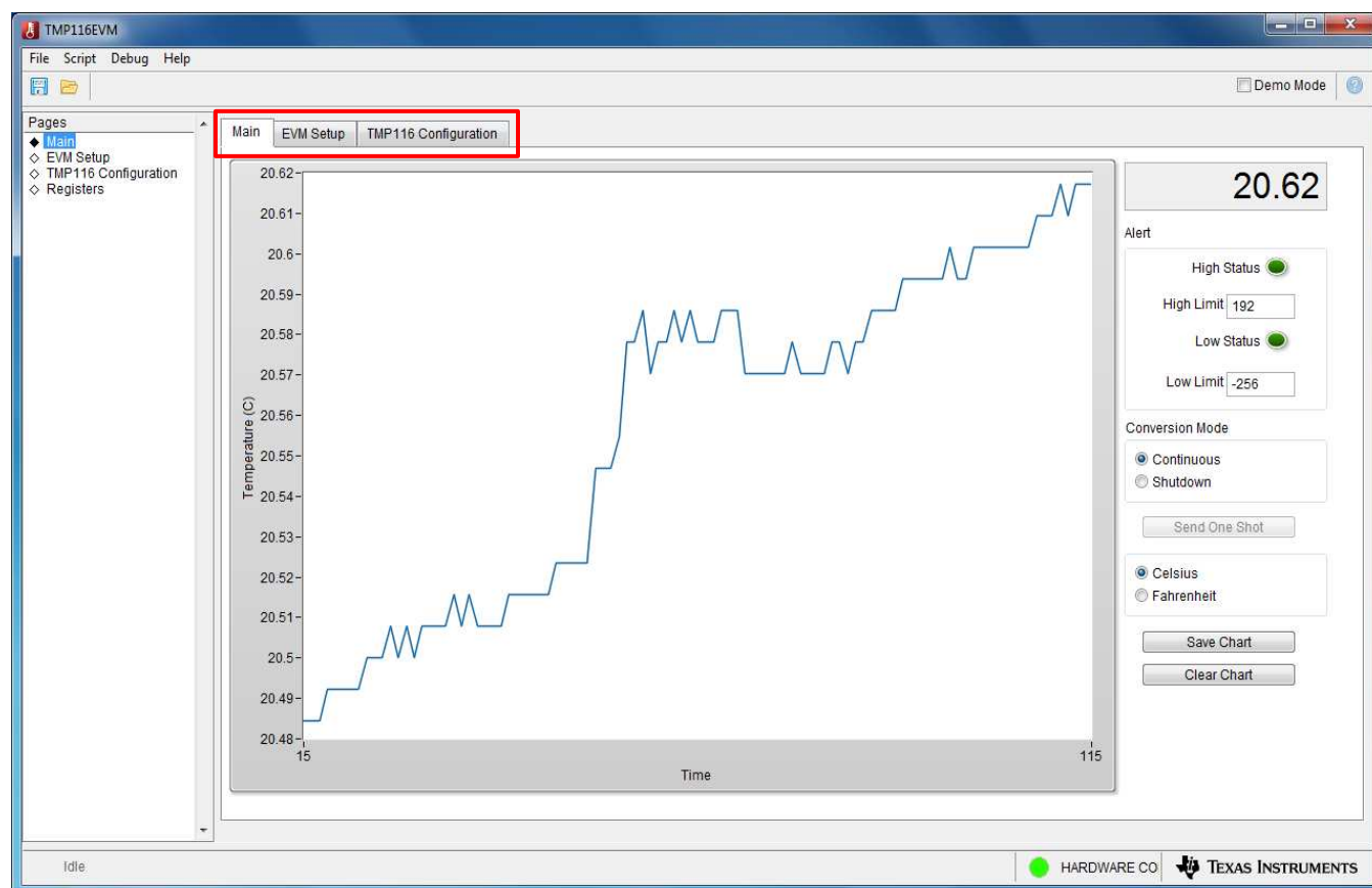
Figure 17. TMP116EVM Default Tab
