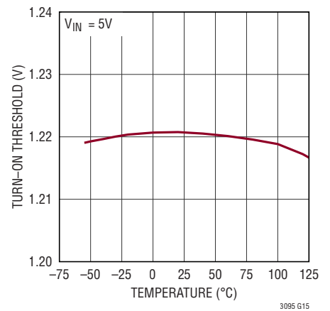
EN Turn-On Threshold
