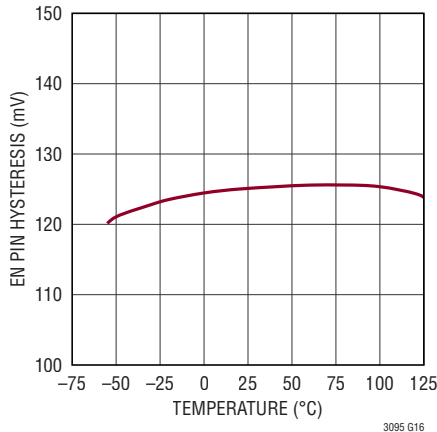
EN Pin Hysteresis
