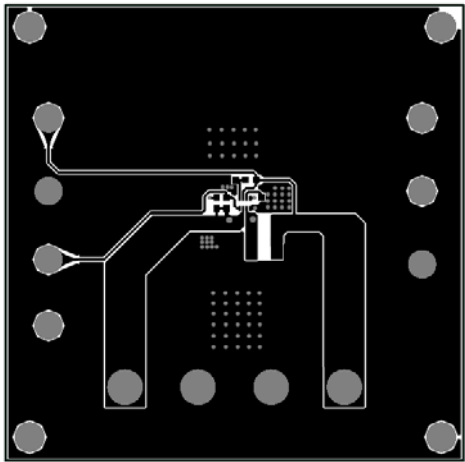
Figure 4—Top Layer
