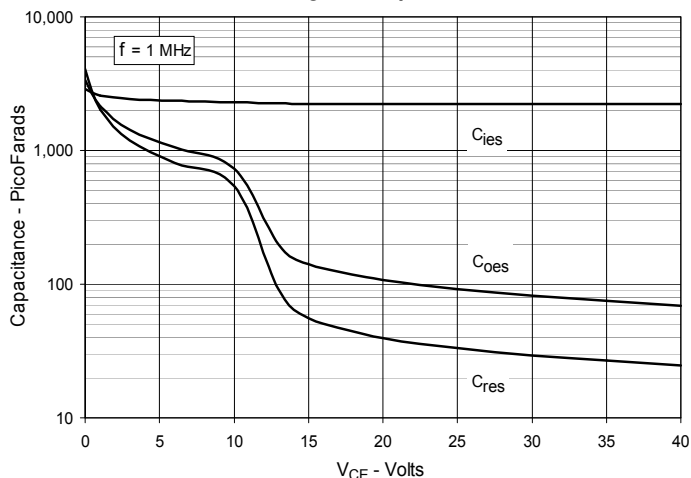
Fig. 10. Capacitance
