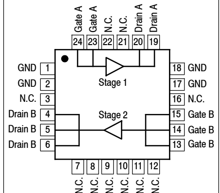
QFN 4 × 4
