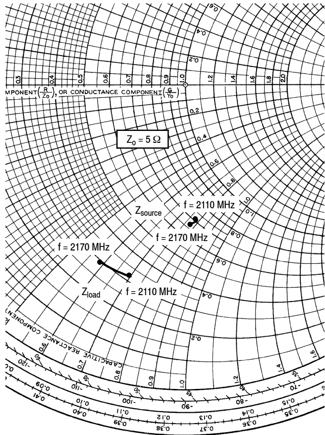
MRF6S21100NBR1
