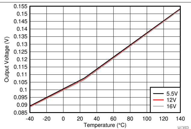
Figure 18. LO Low Output Voltage (V LOL )
