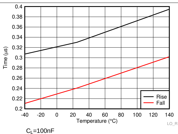
Figure 26. LO Rise & Fall Time
