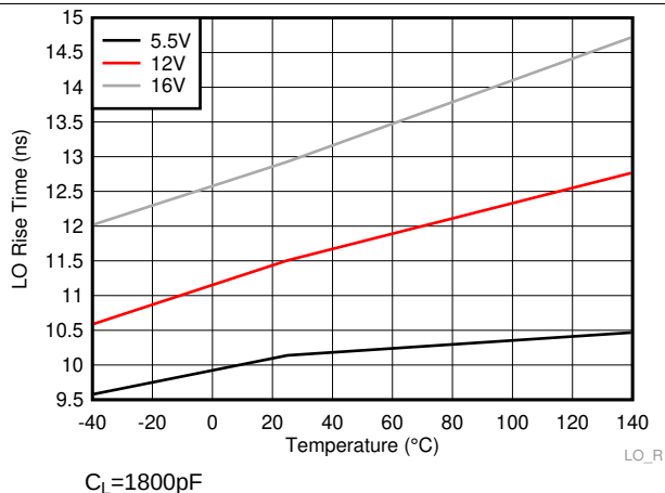
Figure 22. LO Rise Time
