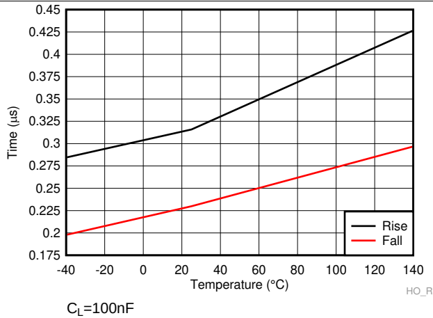
Figure 27. HO Rise & Fall Time
