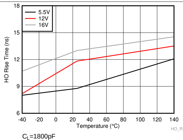
Figure 24. HO Rise Time
