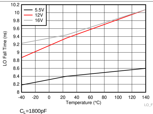
Figure 23. LO Fall Time
