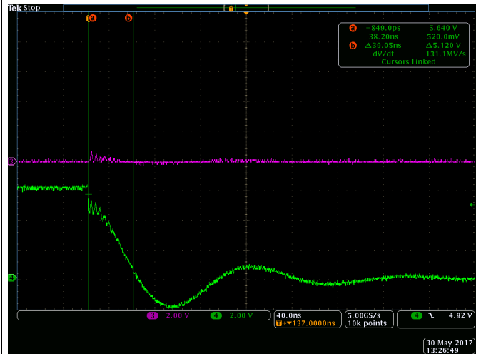
Figure 38. LO Fall Time
